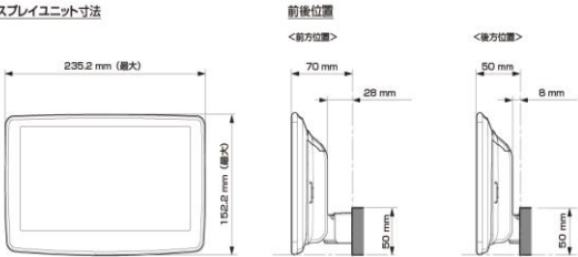
ディスプレイユニット寸法
