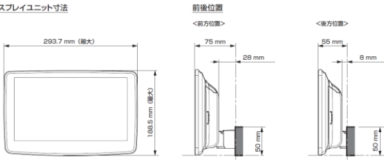
ディスプレイユニット寸法
