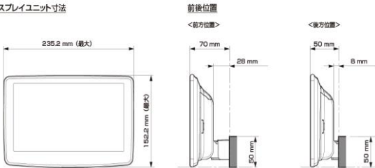
■ ディスプレイ取り付け寸法と調整可能位置
