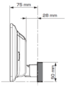
前後位置
