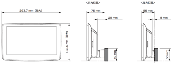
■ ディスプレイ取り付け寸法と調整可能位置
