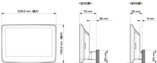
ディスプレイユニット寸法
