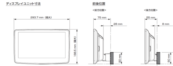
■ ディスプレイ取り付け寸法と調整可能位置
