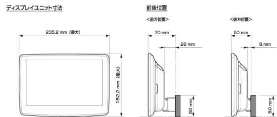
■ ディスプレイ取り付け寸法と調整可能位置
