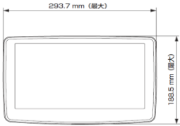
ディスプレイユニット寸法
