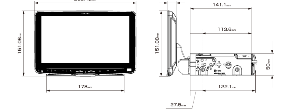
【寸法図】
